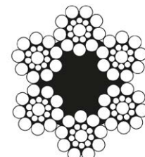
6x19 FC
